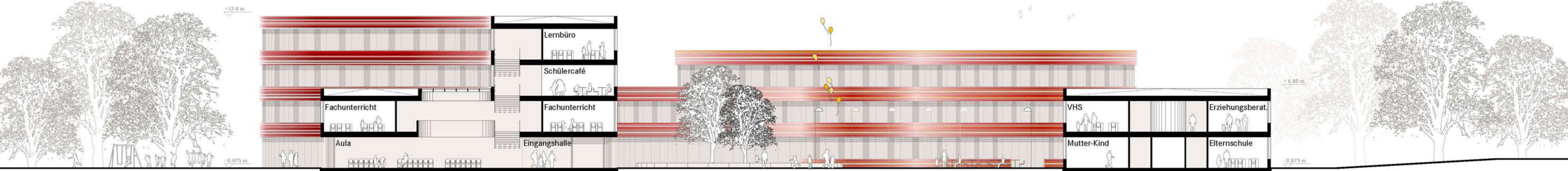
Querschnitt A-A Stadtteilschule - Quartierszentrum M 1:200
